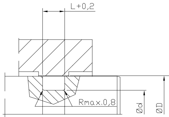
geschlossener Einbauraum
