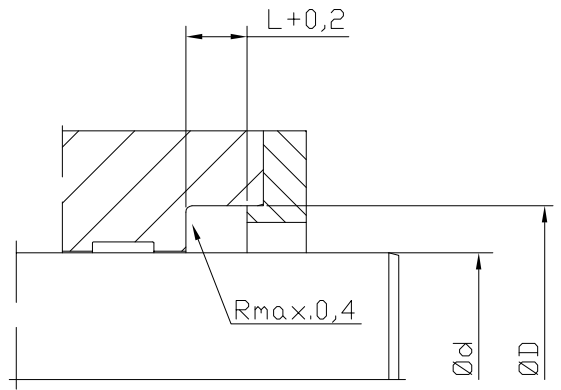
offener Einbauraum
