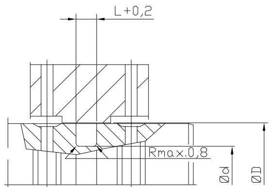
geschlossener Einbauraum
