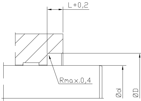
offener Einbauraum
