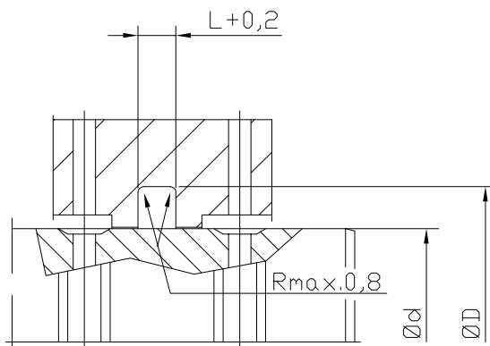
geschlossener Einbauraum
