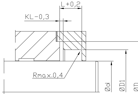
offener Einbauraum
