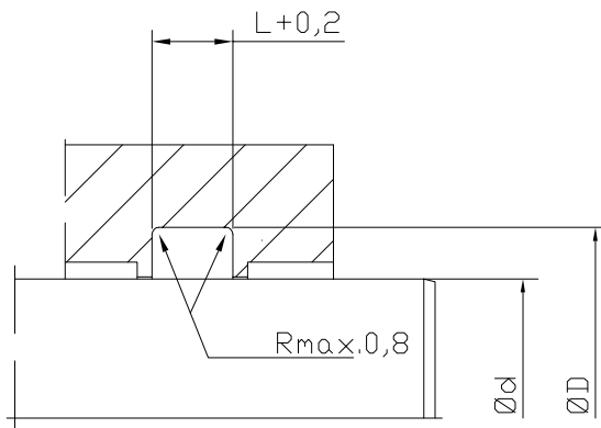
geschlossener Einbauraum
