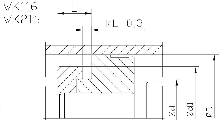
offener Einbauraum
