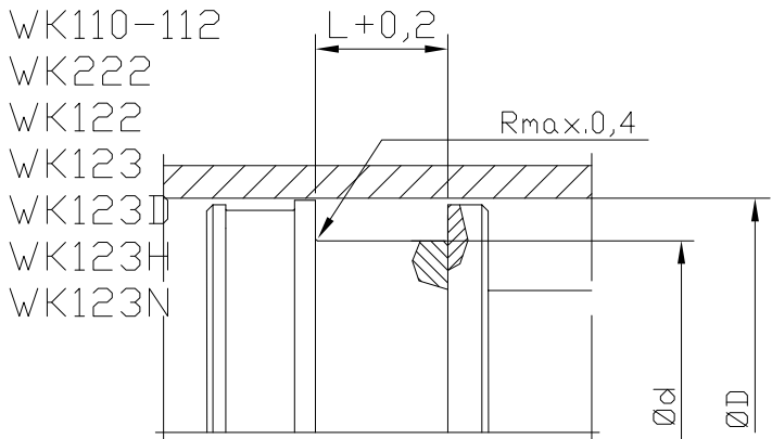
offener Einbauraum
