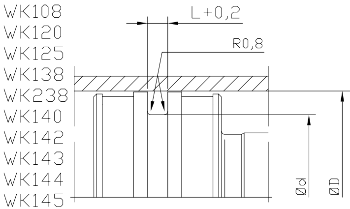
geschlossener Einbauraum
