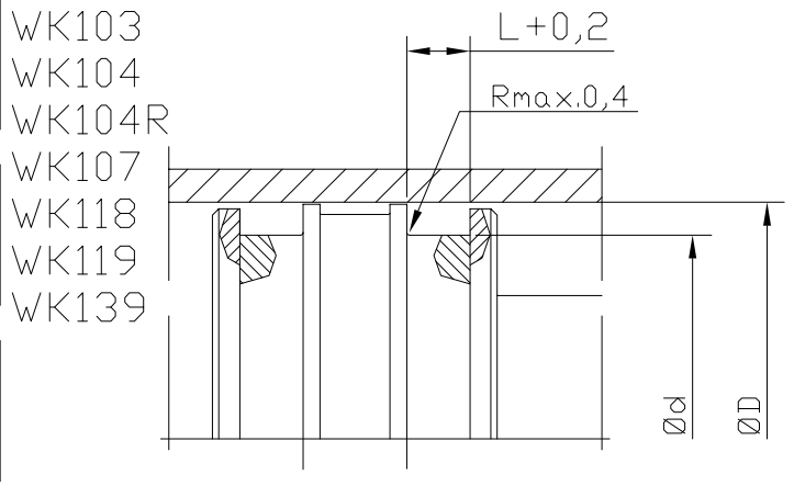
offener Einbauraum
