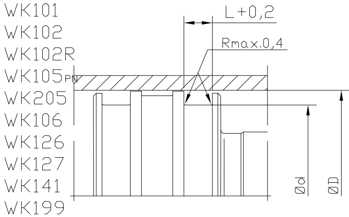
geschlossener Einbauraum
