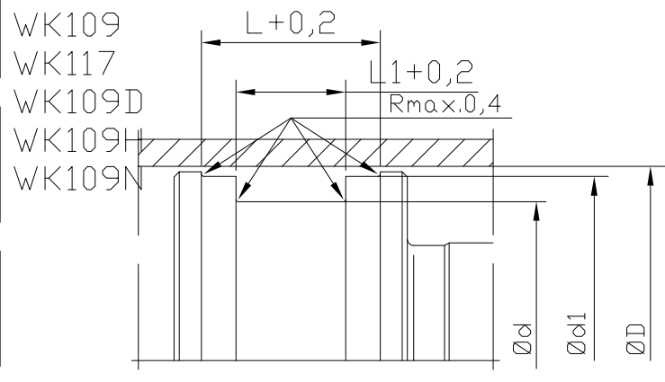
geschlossener Einbauraum
