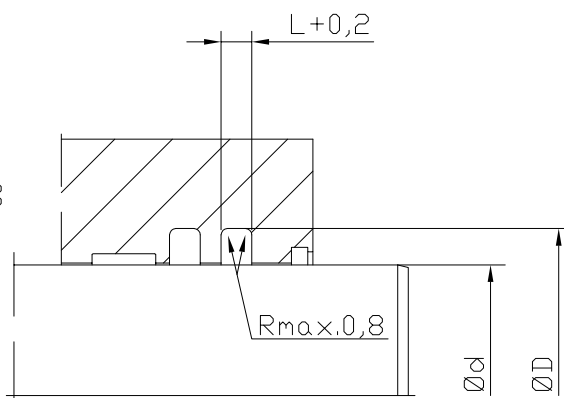
geschlossener Einbauraum
