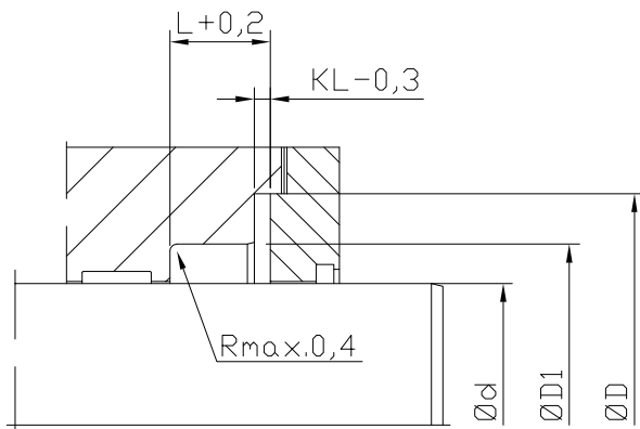
offener Einbauraum
