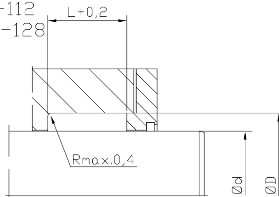
offener Einbauraum
