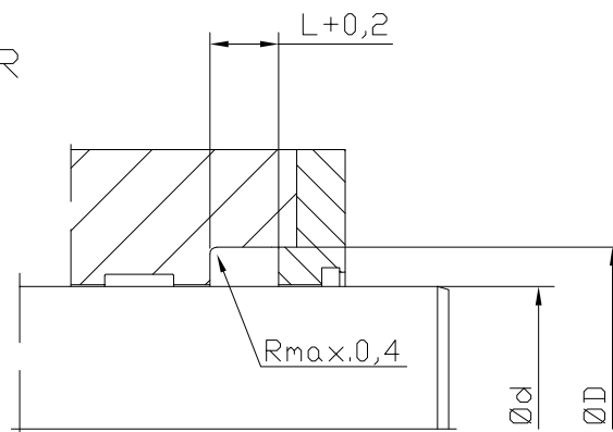
offener Einbauraum
